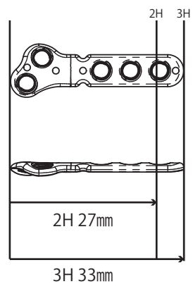
近位/骨幹部用 PM0
